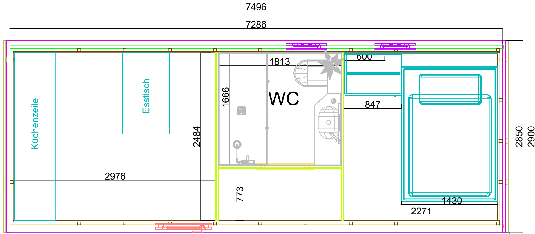
Grundriss Modularer Camping CUBE mit WC, Küche & großer Schlafraum Maße: 247 x 750 x 290cm
